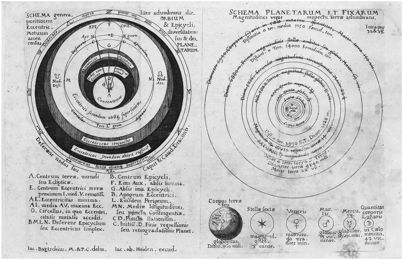
Schéma des orbites planétaires, dans "Usus astronomicus planisphaerii stellati seu vice-globi coelestes"
